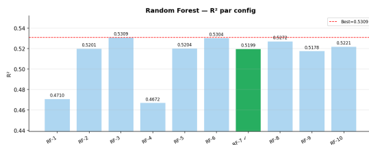
FIGURE 16 – Random Forest - Impact des hyperparamètres
