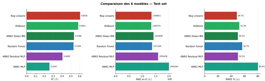
FIGURE 15 – Comparaison des performances des 6 modèles ( R^2 , MAE, MAPE)
