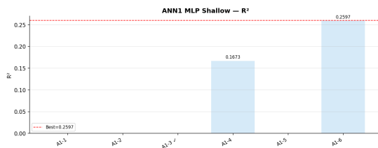
FIGURE 18 – ANN1 MLP Shallow - Impact des hyperparamètres
