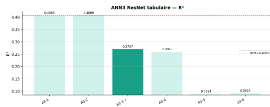
FIGURE 20 – ANN3 Residual MLP - Impact des hyperparamètres
