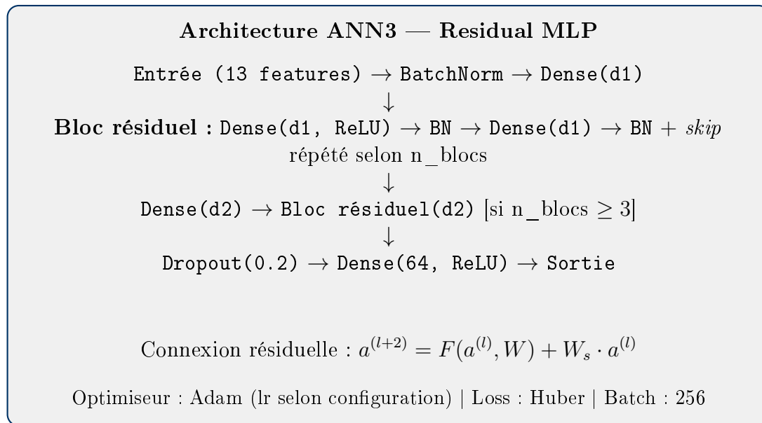
FIGURE 13 – Architecture MLP résiduel pour données tabulaires (ANN3)
