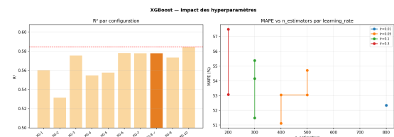
FIGURE 17 – XGBoost - Impact des hyperparamètres
